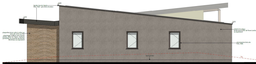
FAÇADE OUEST 1/50 ème
